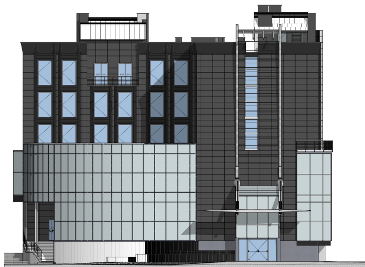
ELEWACJA POŁUDNIOWO WSCHODNIA 1 : 250
